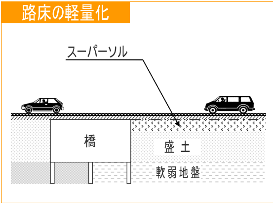
▲モデル図
