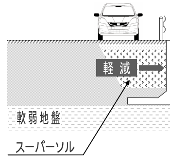
軟弱地盤上のL字よう壁の裏込め
